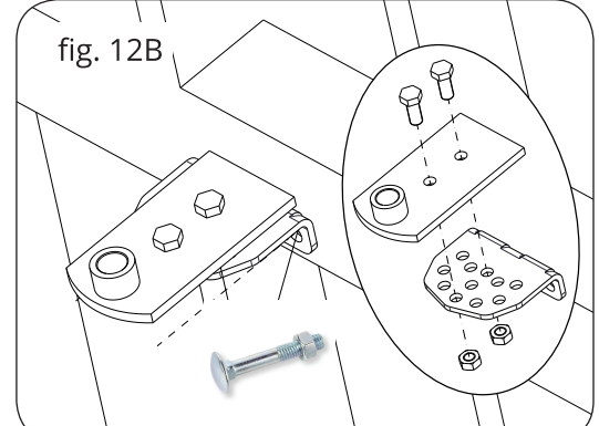
Infästning i ram - Genomgående Vangsbult
