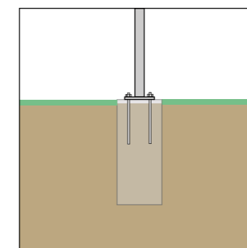
Fotplatta: Stolpen monteras med gängstänger/expanderbult på plint/platta.
