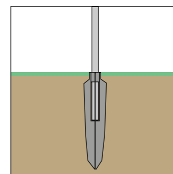
Stolpankare: Stolpen monteras i stolpankare som drivits ner i marken.
